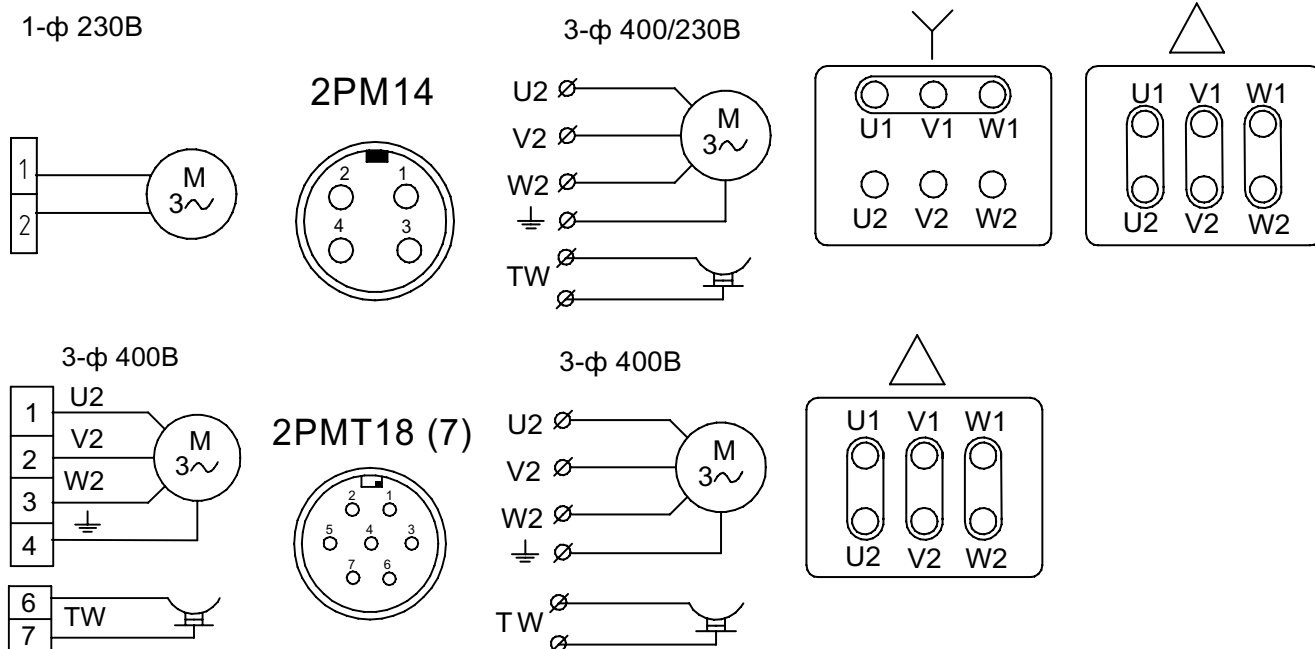
Рис. 26 Схема подключения вентилятора принудительной вентиляции.
