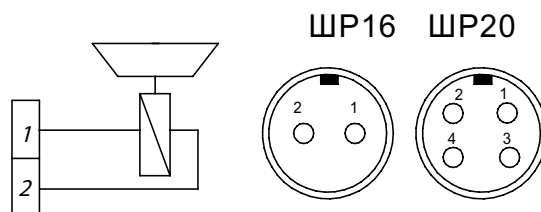
Рис. 25 Схема подключения электромагнитного тормоза.
