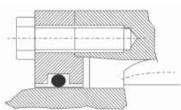
Вид X для муфты зубчатой от размера 111 и выше
